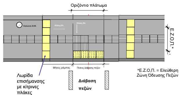
Ράμπα σε πεζοδρόμιο ύψους 8εκ.
