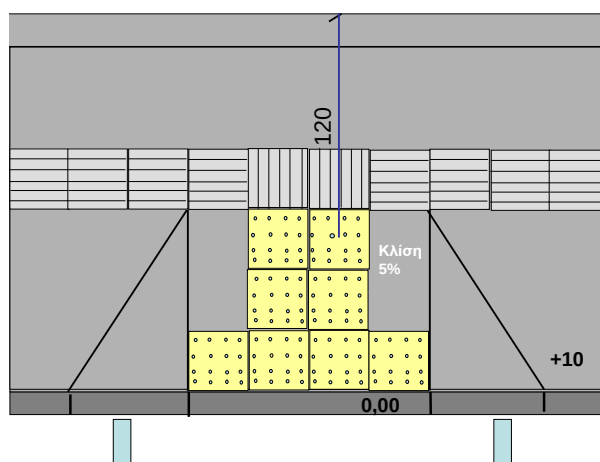
Ράμπα κάθετη προς πεζοδρόμιο ύψους 8-10εκ. με οριζόντιο πλάτωμα 1,20μ. στο πάνω μέρος.
